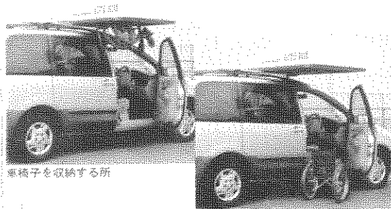
展開して車椅子を吊上げる所
